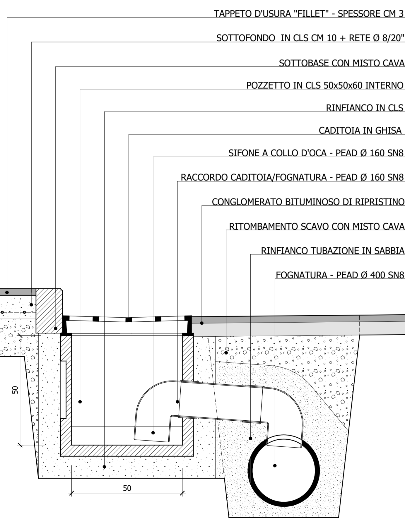
SEZIONE TIPO CADITOIA 1/10
